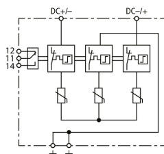
Esquema del DCB YPV 1200 FM
