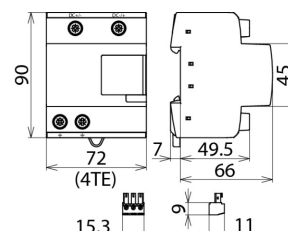
Dimensiones del DCB YPV 1200 FM
