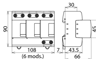
Dimensiones del DV M TNC 255
