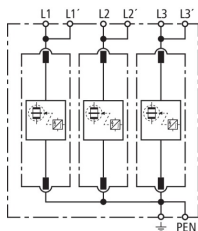
Esquema del DV M TNC 255
