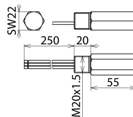
Dimensiones del DPI CD EXD 24 M
